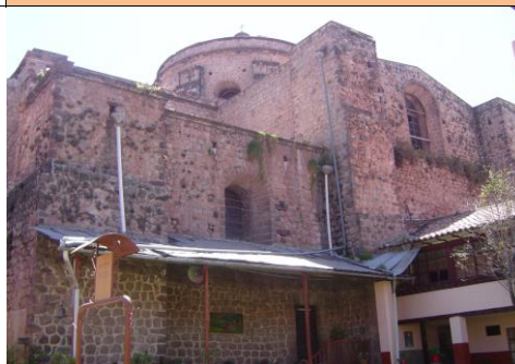
F17 VISTA FRONTISPICIO EN MURO DEL EVANGELIO
