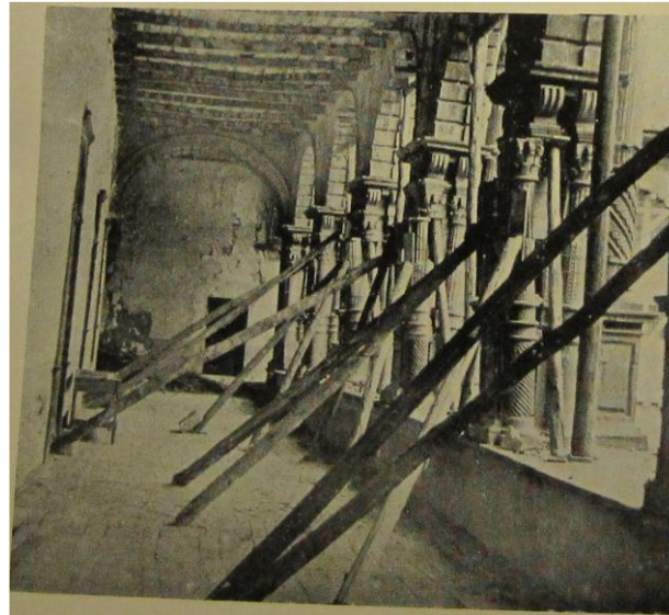
Apuntalamiento de las Pilastras de los altos del primer claustro del Convento.
